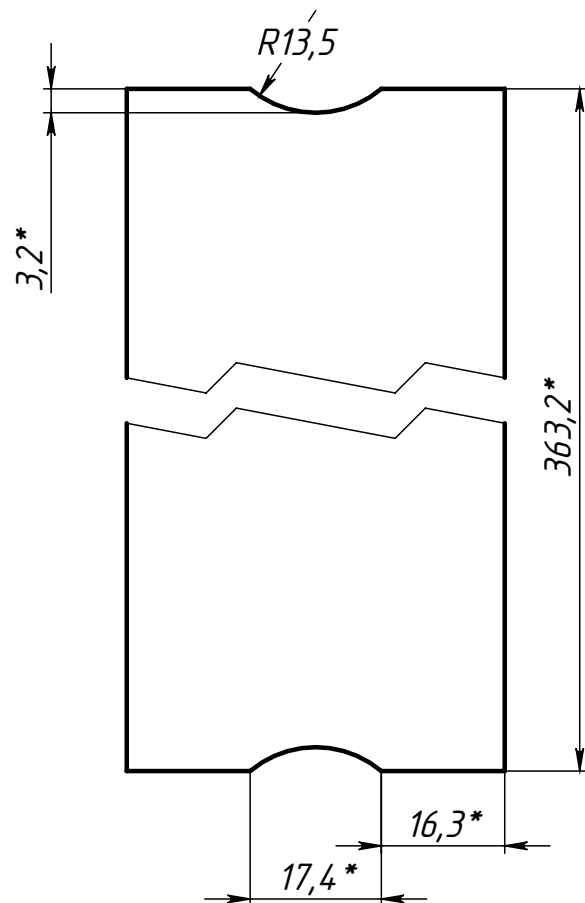
Поз.1 (Корпус) 1 : 1
